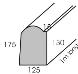
Modcon Kerbing Type 009
