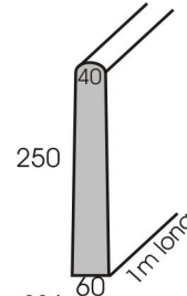
Modcon Kerbing Type 004
